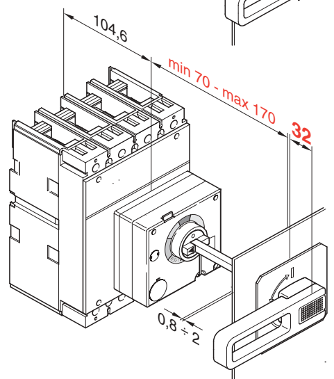
D - IP40
