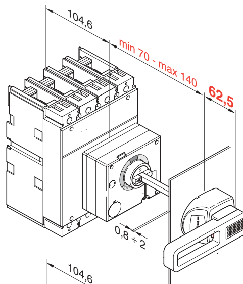
A - IP55
